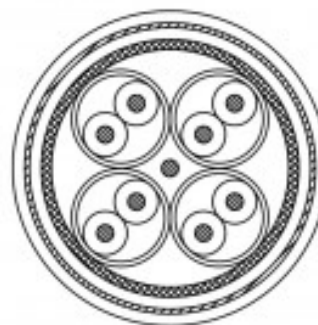
Sección transversal
